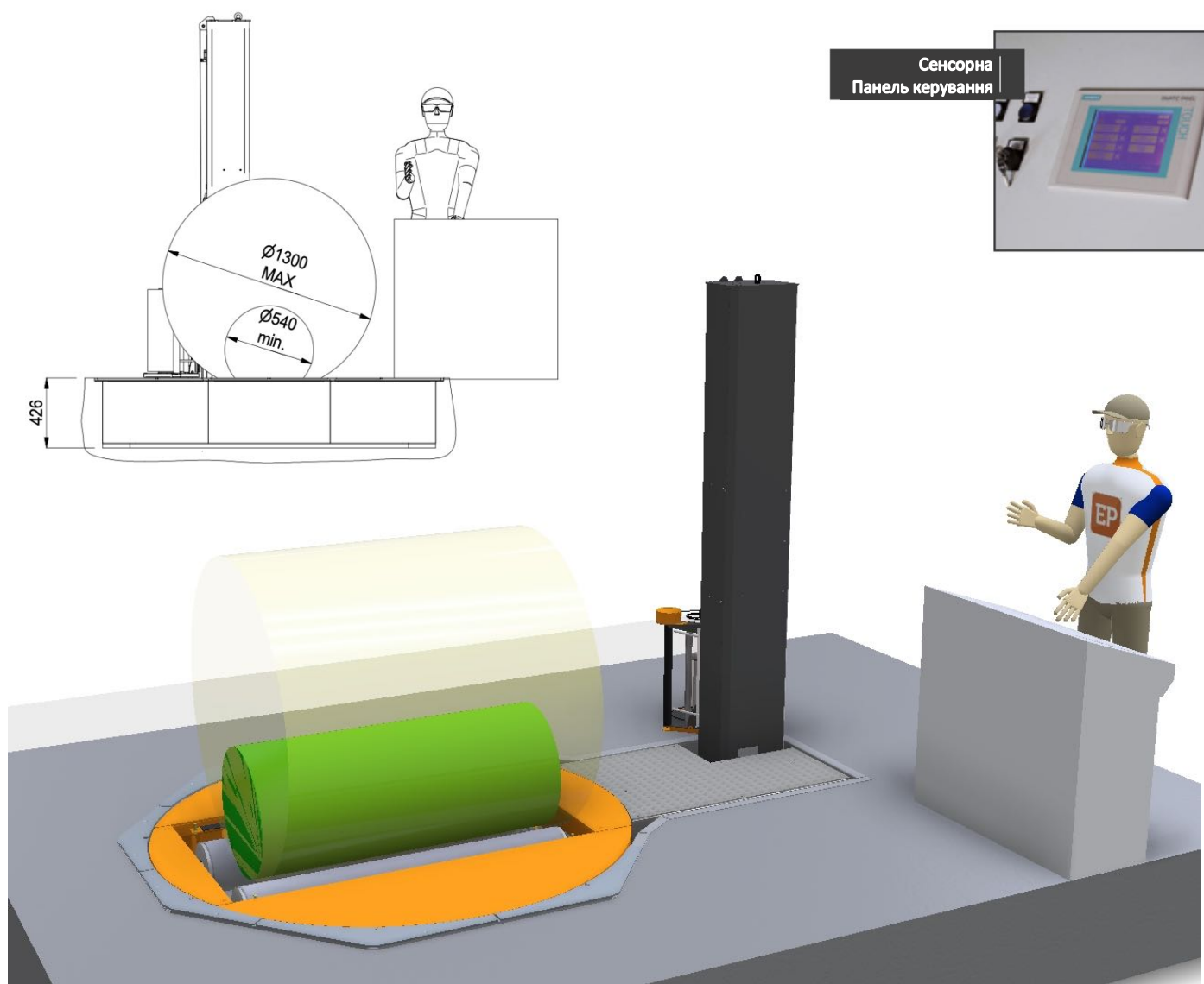
Платформний палетообмотувач PLUS SPECIALE 2000
